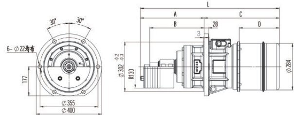
图3 侧板振动电机外形安装图 (SIZE90 91 A)
